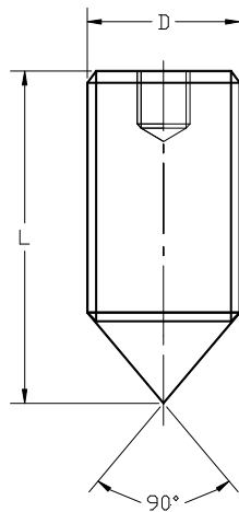
DIN 914 1803
