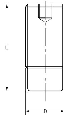
DIN 915 1804
